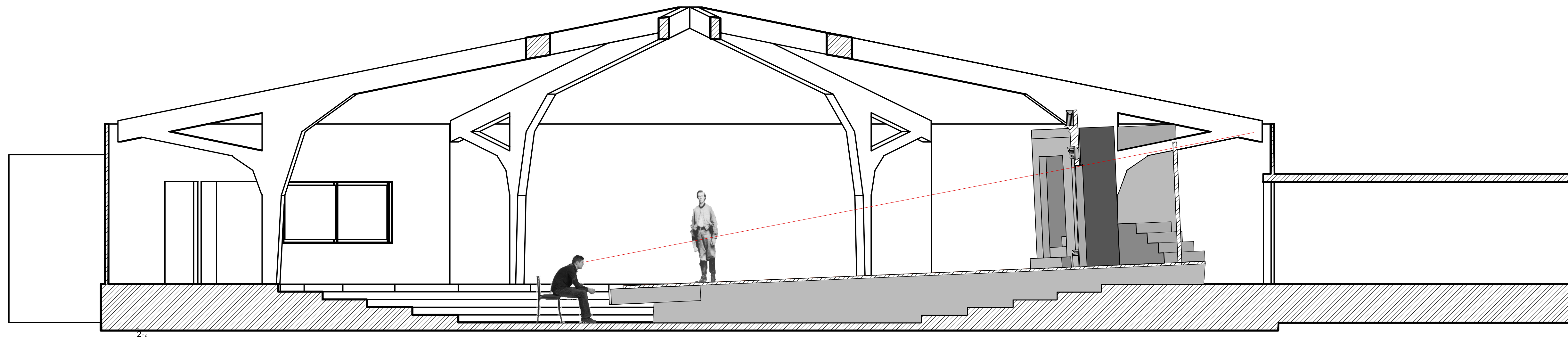
1 SECTION Scale: 1/4" = 1'-0"
