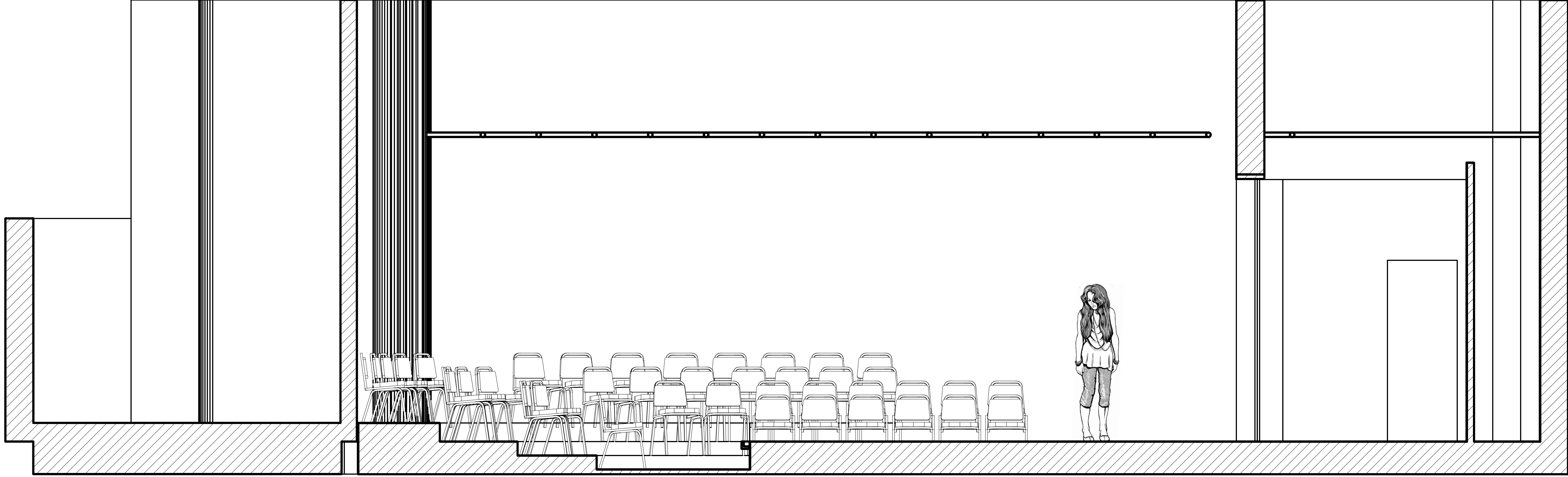
1 CENTERLINE SECTION Scale: 1/2" = 1'-0"
